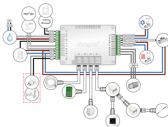
Figure 5. Régulateur URC1.
